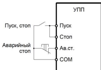
Рисунок 5 – Трехпроводная и двухпроводная схема управления
